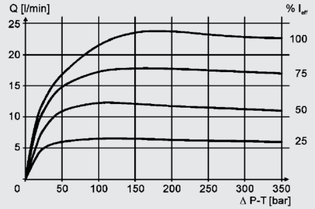
Q 16 spool
