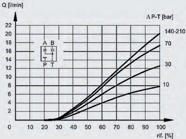
Q 08 spool
