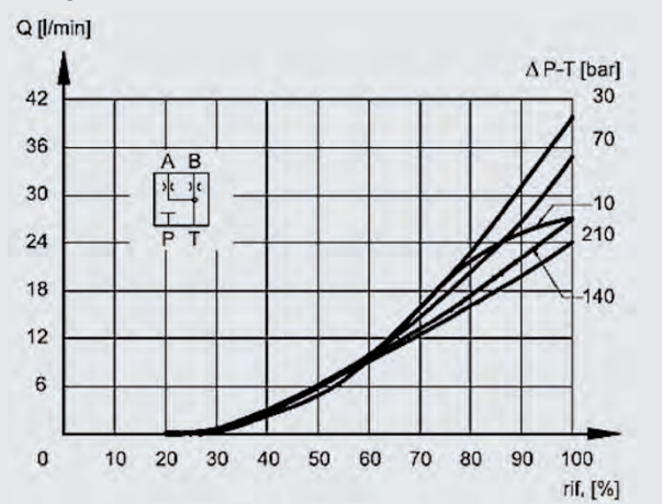
Q 26 spool
