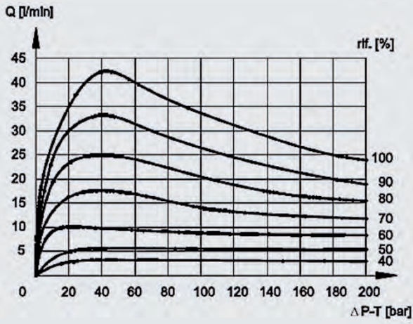
Q 04 spool
