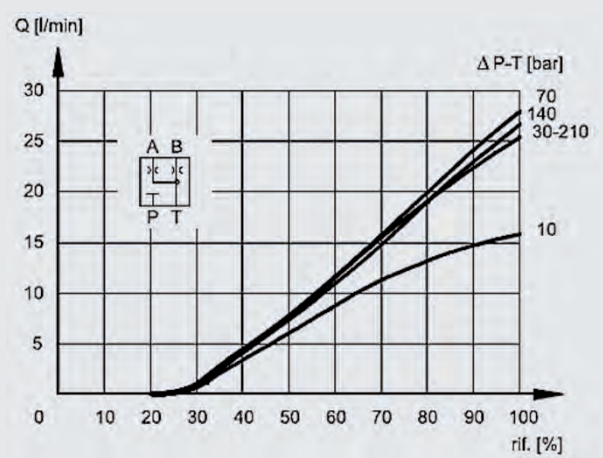
Q 16 spool
