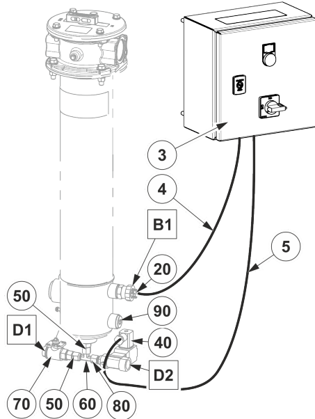
Abb. 1: Funktionsprinzip des AWD am LVH-CD-118 vertikal
