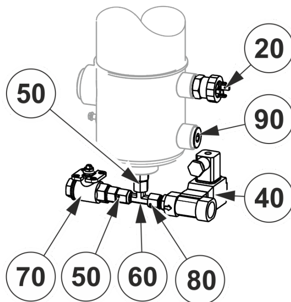
Abb. 5: Hydraulische Installation
