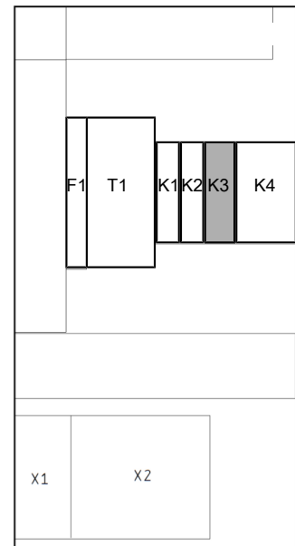
Abb. 6: Schaltschrank, Innenansicht
